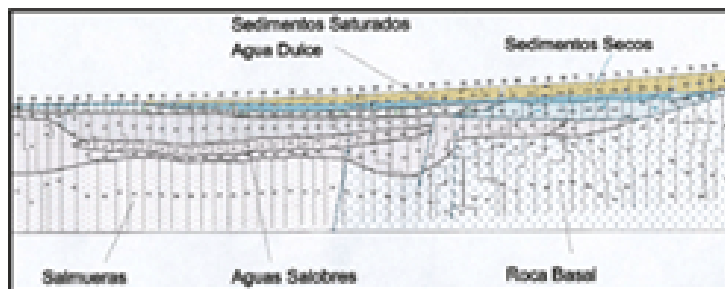
Sección Geofísica TEM
